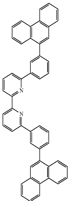
[Chem 9]
