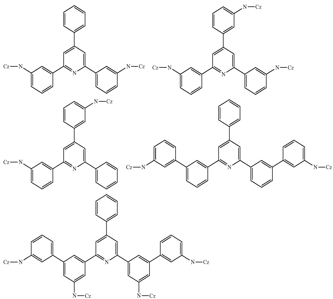
[Chem 9]
